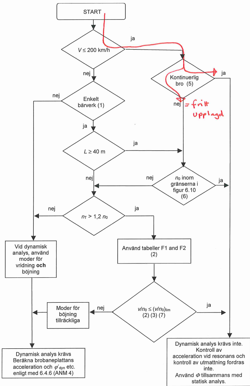
Figur 6.9 – Flödesschema för att avgöra om dynamisk analys erfordras
